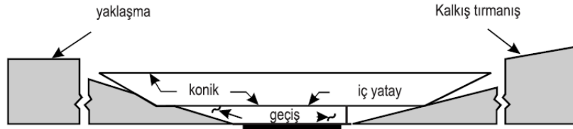
A-A Kesiti
