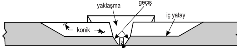
B-B Kesiti
