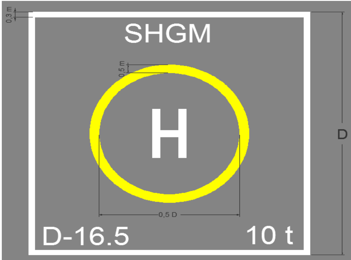
Şekil 3-5. Heliport İşaretlemeleri (Örnek)
