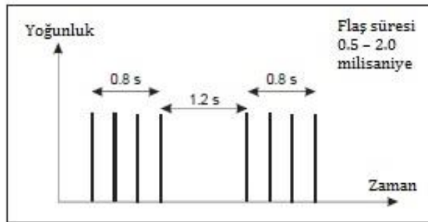
Şekil 3-10. Heliport bikını flaş özellikleri
