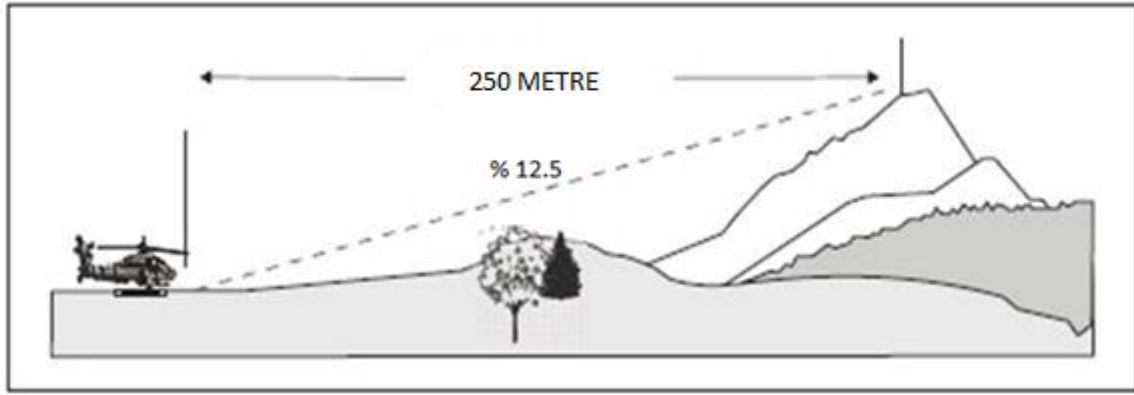
Şekil 2-1. Mânia Sınırlama Yüzeyleri
