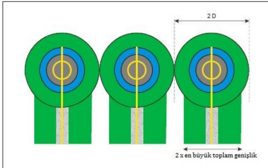
Şekil 1-5. Hava taksit güzergahları/taksit yolları ile hover dönüşler için tasarlanmış olan helikopter park yerleri – eş zamanlı operasyonlar
