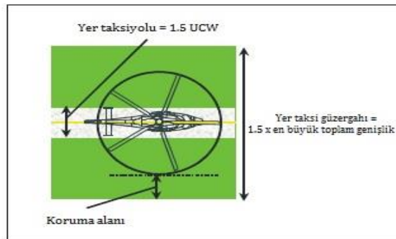
Şekil 1-2 Helikopter yer taksi güzergahı / taksiyolu
