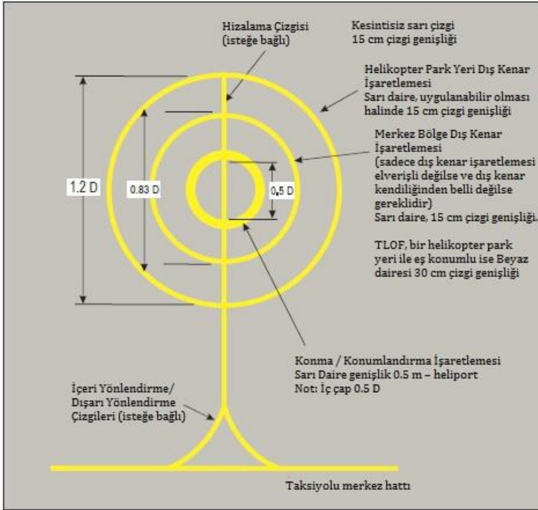
Şekil 3-7. Helikopter park yeri işaretlemeleri
