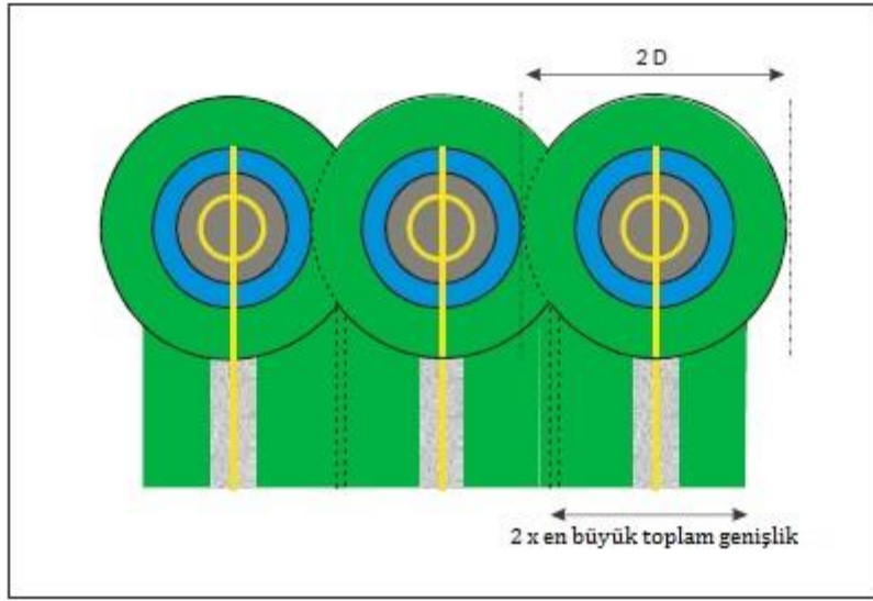
Şekil 1-6. Hava taksi güzergahları/taksi yolları ile hover dönüşler için tasarlanmış olan helikopter park yerleri1– eş zamanlı olmayan operasyonlar
