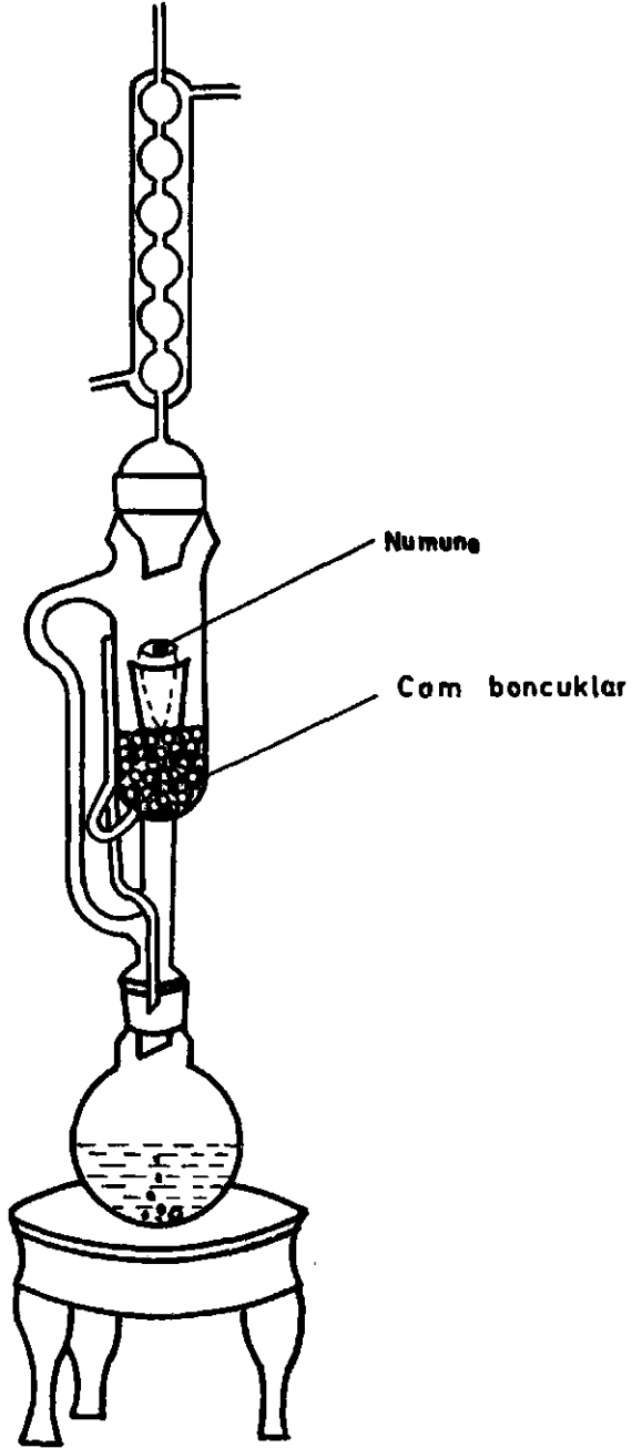
ŞEKİL 2. Alkolde çözünmeyen maddelerin tayin cihazı
