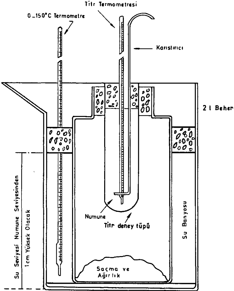
ŞEKİL-5 TİTR DENEY CİHAZI
