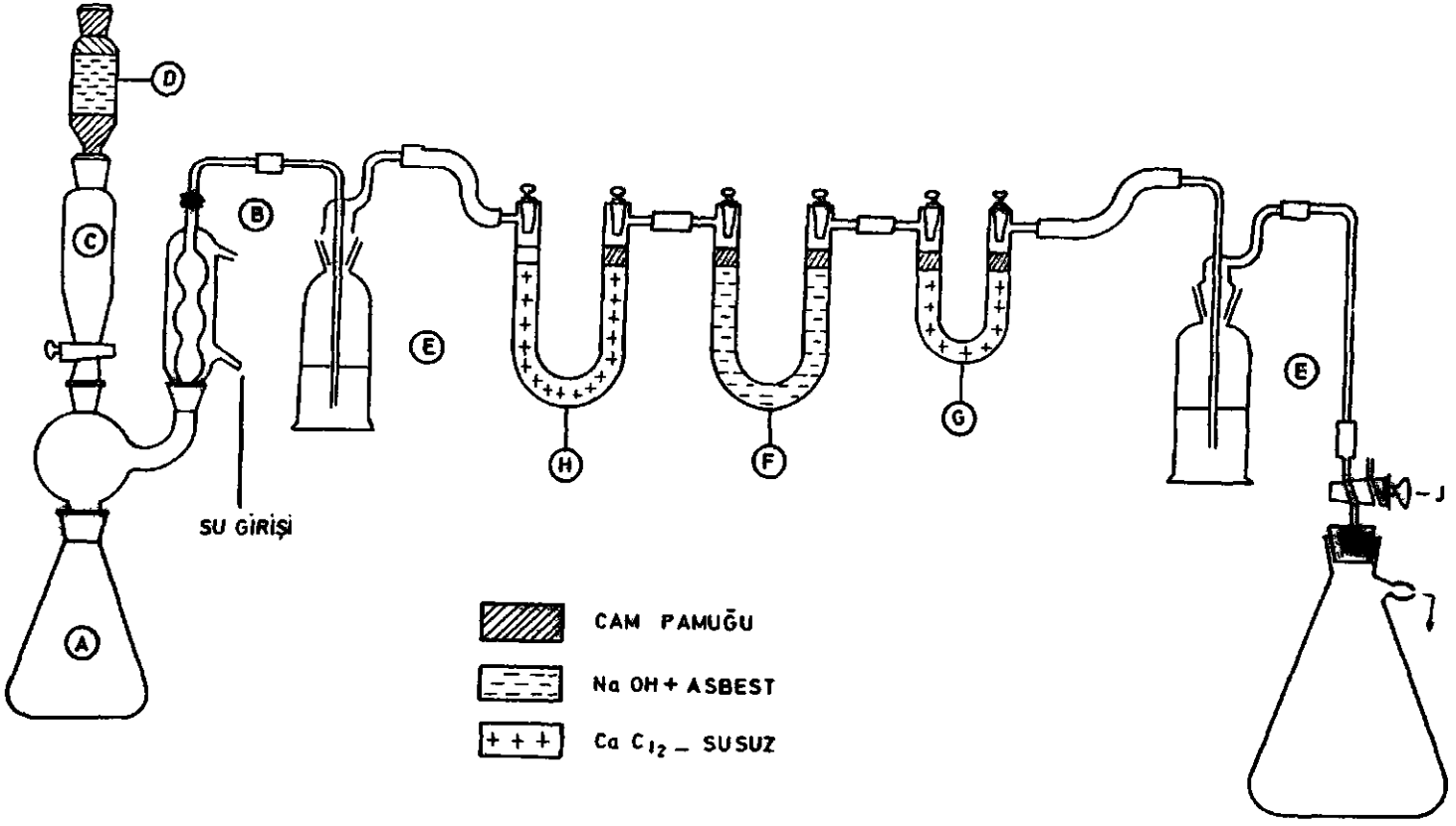
ŞEKİL 4 - KARBONAT MİKTARI TAYİN CİHAZI
