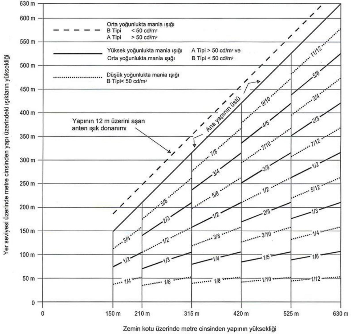
Şekil A6-7. Yüksek/orta yoğunlukta ikili mânia ışıklandırma sistemi, Tip A/Tip B
