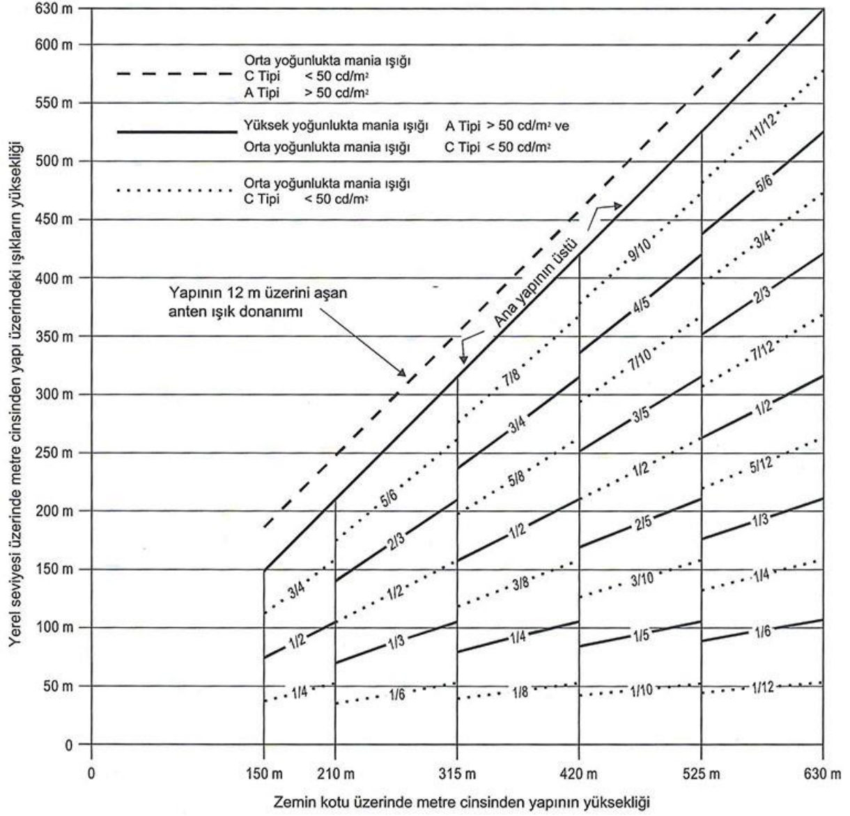
Şekil A6-8. Yüksek/orta yoğunlukta ikili mânia ışıklandırma sistemi, Tip A/Tip C
