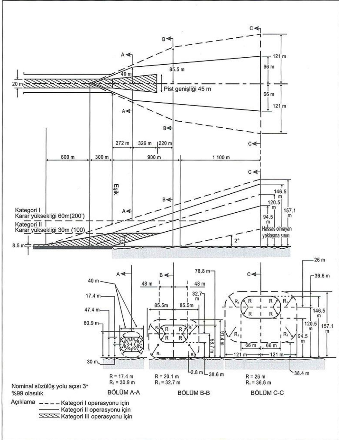
Şekil A-6. Kategori I, II ve III operasyonları için ışılandırma tasarımı için kullanılacak uçuş yolu sargıları
