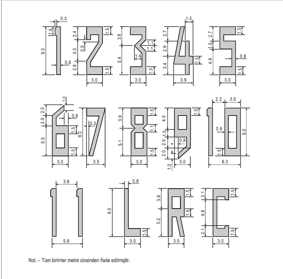
Şekil 5-3. Pist tanıtma işaretlemelerine yönelik rakamların ve harflerin şekil ve orantıları
