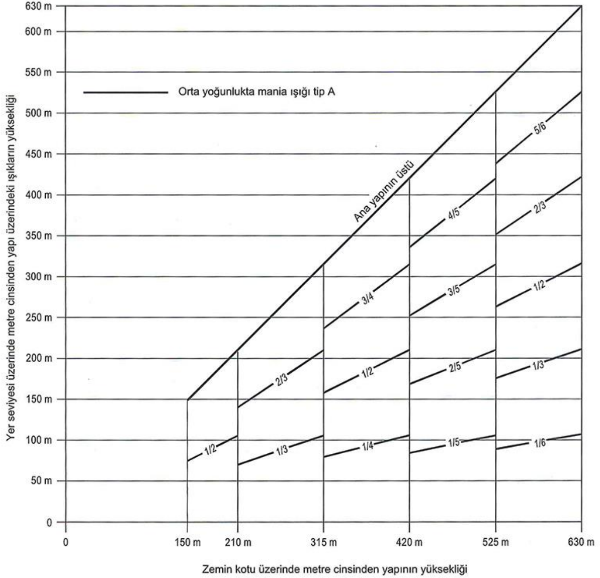
Şekil A6-6. Yüksek yoğunlukta yanıp sönen beyaz mânia ışıklandırma sistemi, Tip A
