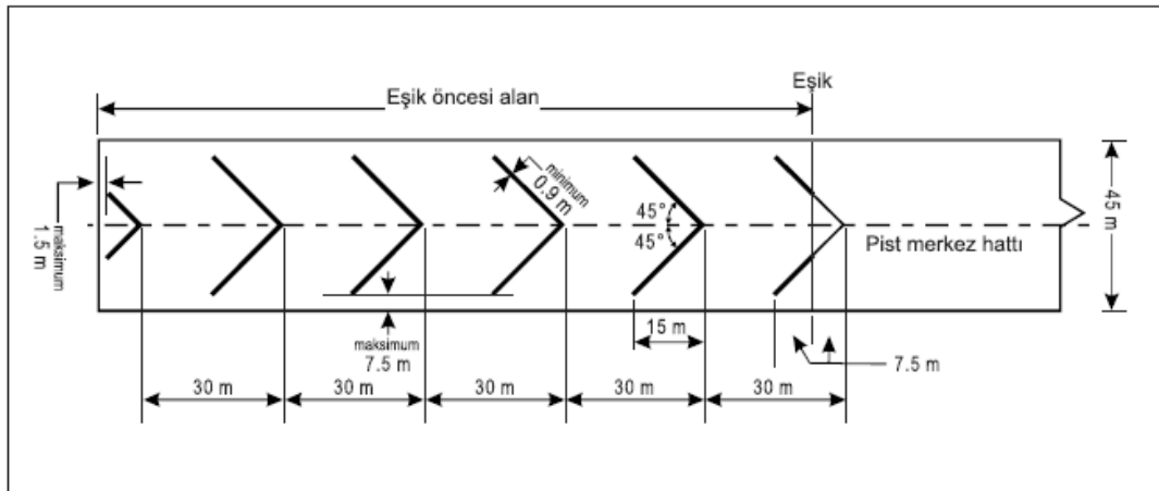
Şekil 7-2. Eşik öncesi işaretleme
