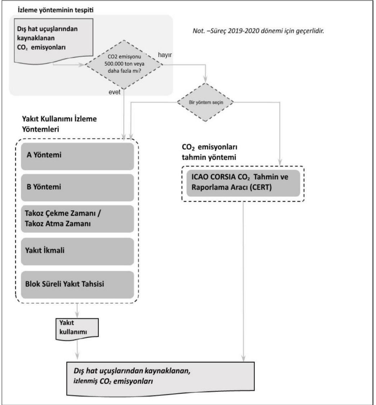
Şekil 12-2. 2019-2020 dönemi boyunca Yakıt Kullanımı İzleme Yöntemlerinin uygunluğuna ilişkin süreç
