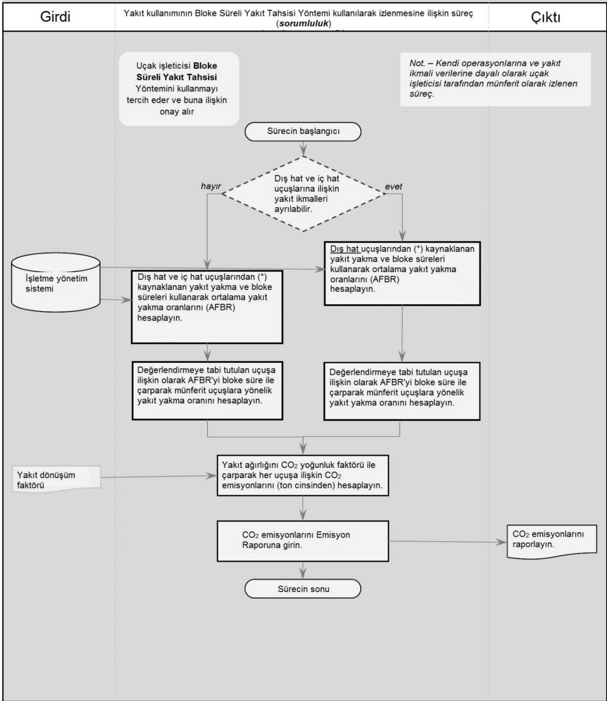
Şekil 13-8. Blok süre/uçuş süresi ile yakıt tahsisi yöntemi kullanılarak uçuş bazında gerçekleştirilen yakıt kullanımının izlenmesine ilişkin süreç
