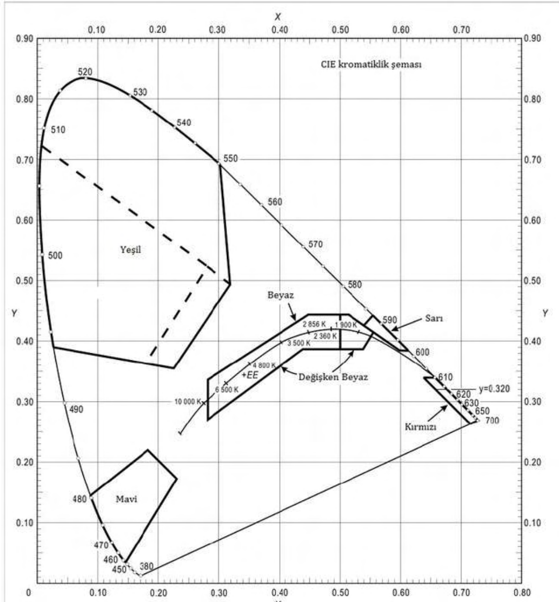
Şekil A1-1a. Havacılık yer ışıklarının renkleri (flamanlı lambalar)
