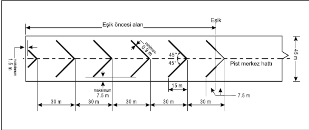
Şekil 7-2. Eşik öncesi işaretleme
