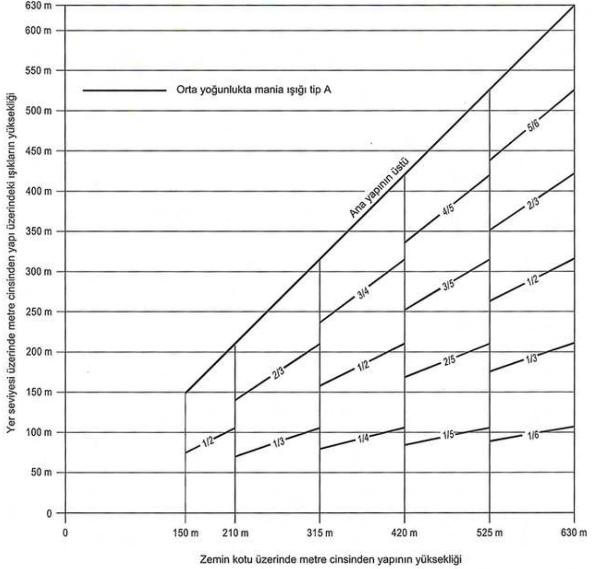
Şekil A5-6. Yüksek yoğunlukta yanıp sönen beyaz mania ışıklandırma sistemi, Tip A
