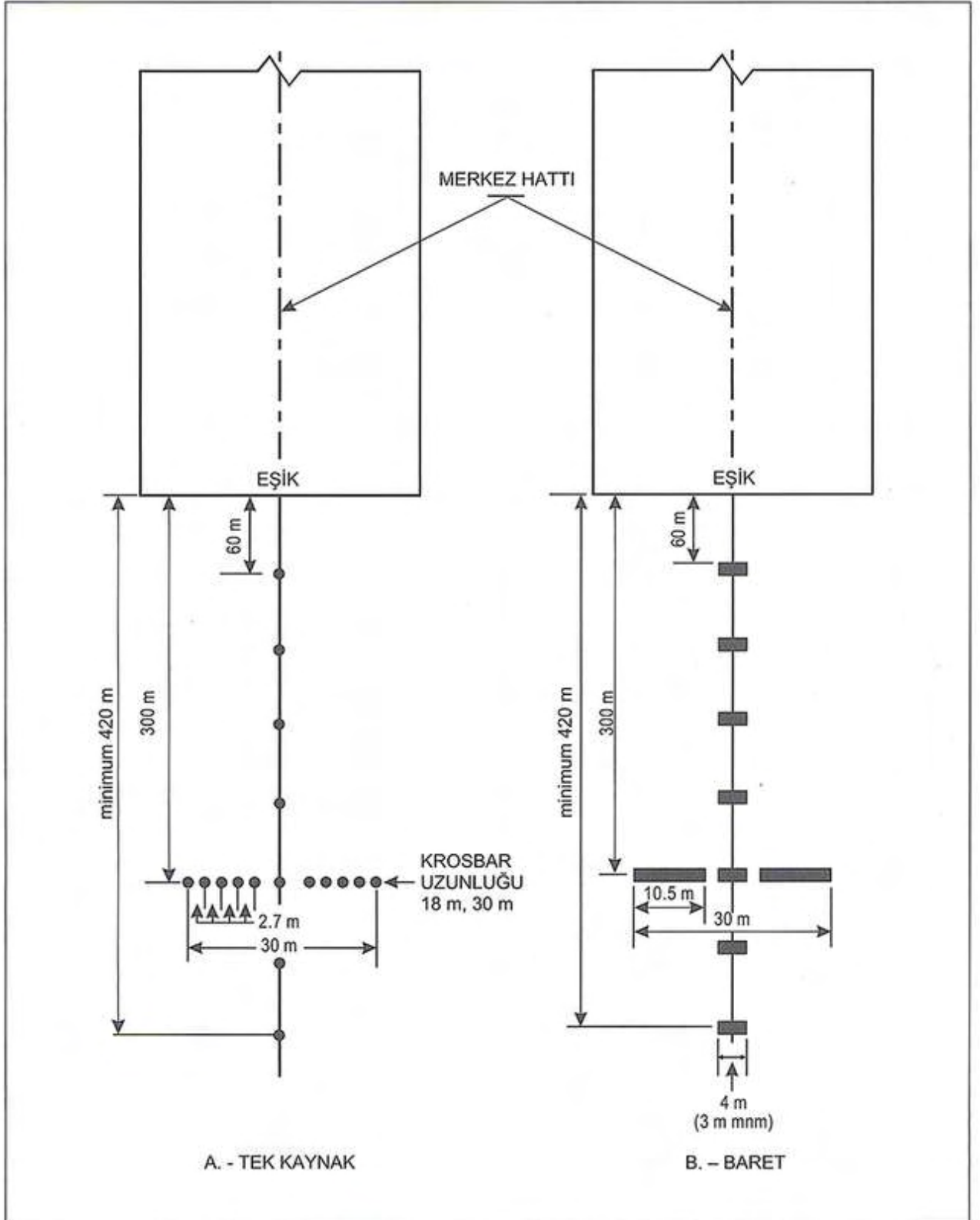
Şekil A-7. Basit yaklaşma ışıklandırma sistemleri
