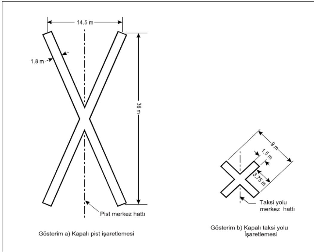
Şekil 7-1. Kapalı pist ve taksi yolu işaretlemeleri
