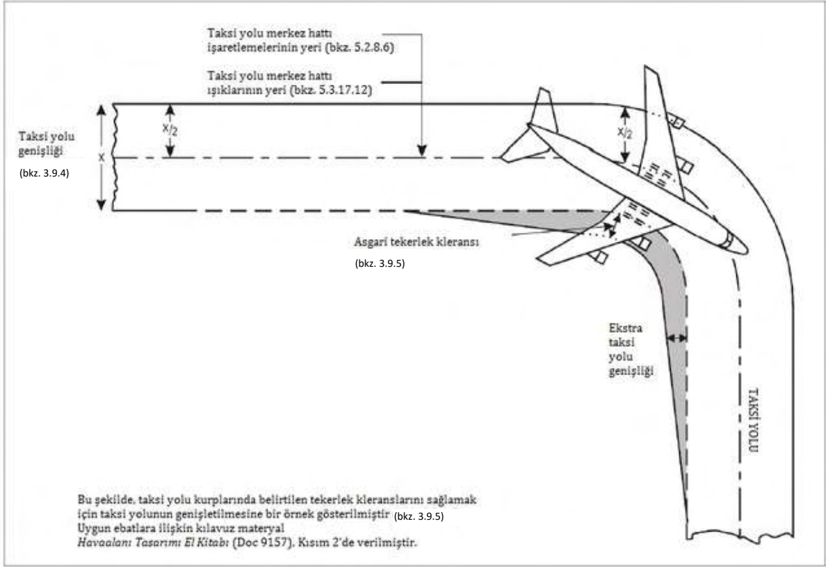
Şekil 3.2. Taksi yolu kurbu
