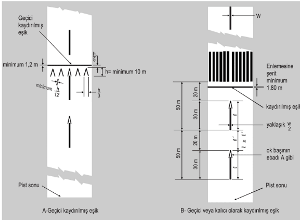
Şekil 5-4. Kaydırılmış Eşik İşaretlemesi
