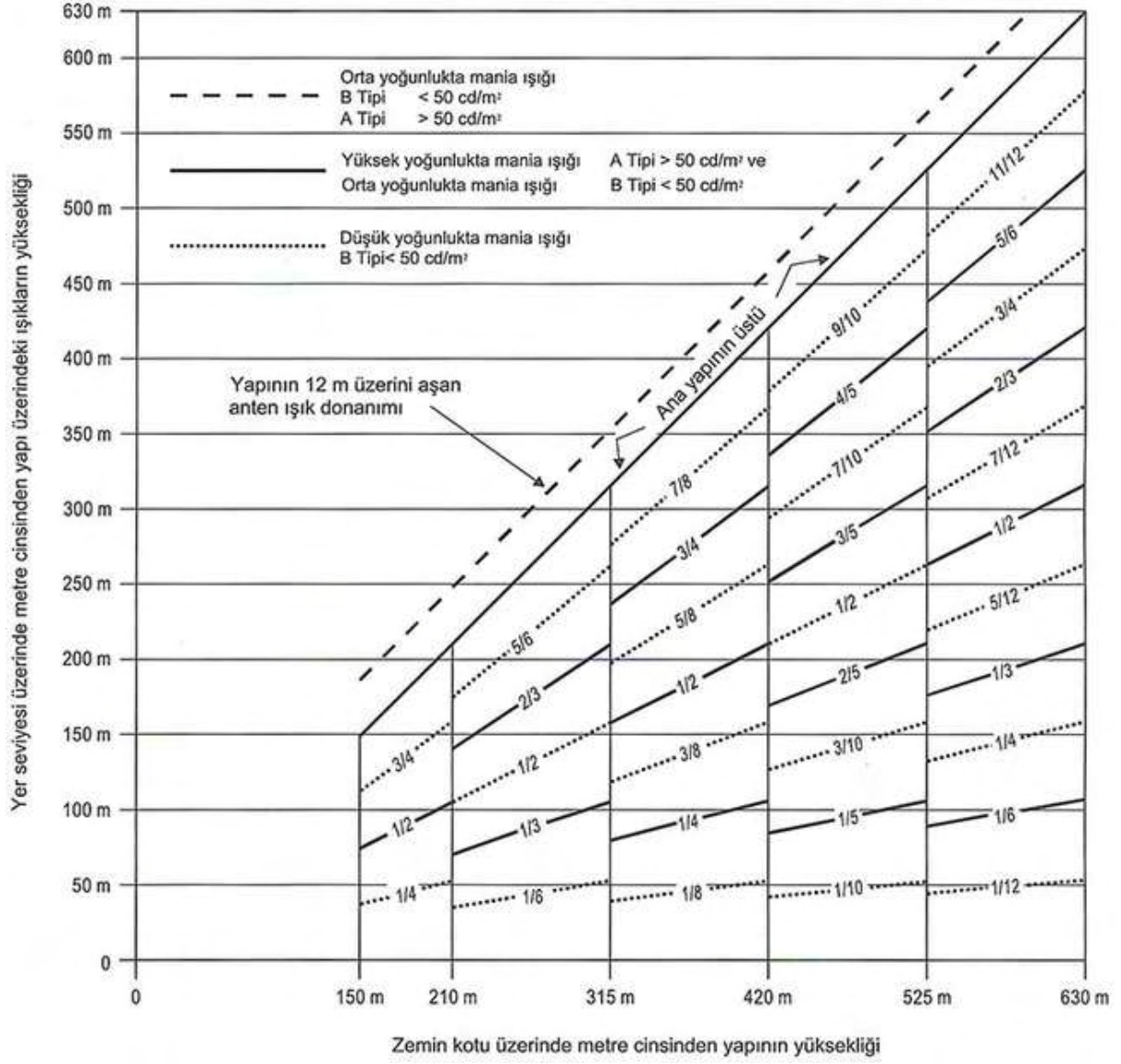
Şekil A5-7. Yüksek/orta yoğunlukta ikili mânia ışıklandırma sistemi, Tip A/Tip B
