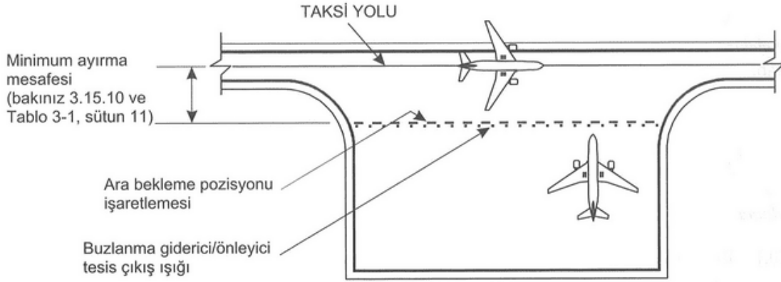
Şekil 5-28 Tipik uzak buzlanma giderici / önleyici tesis
