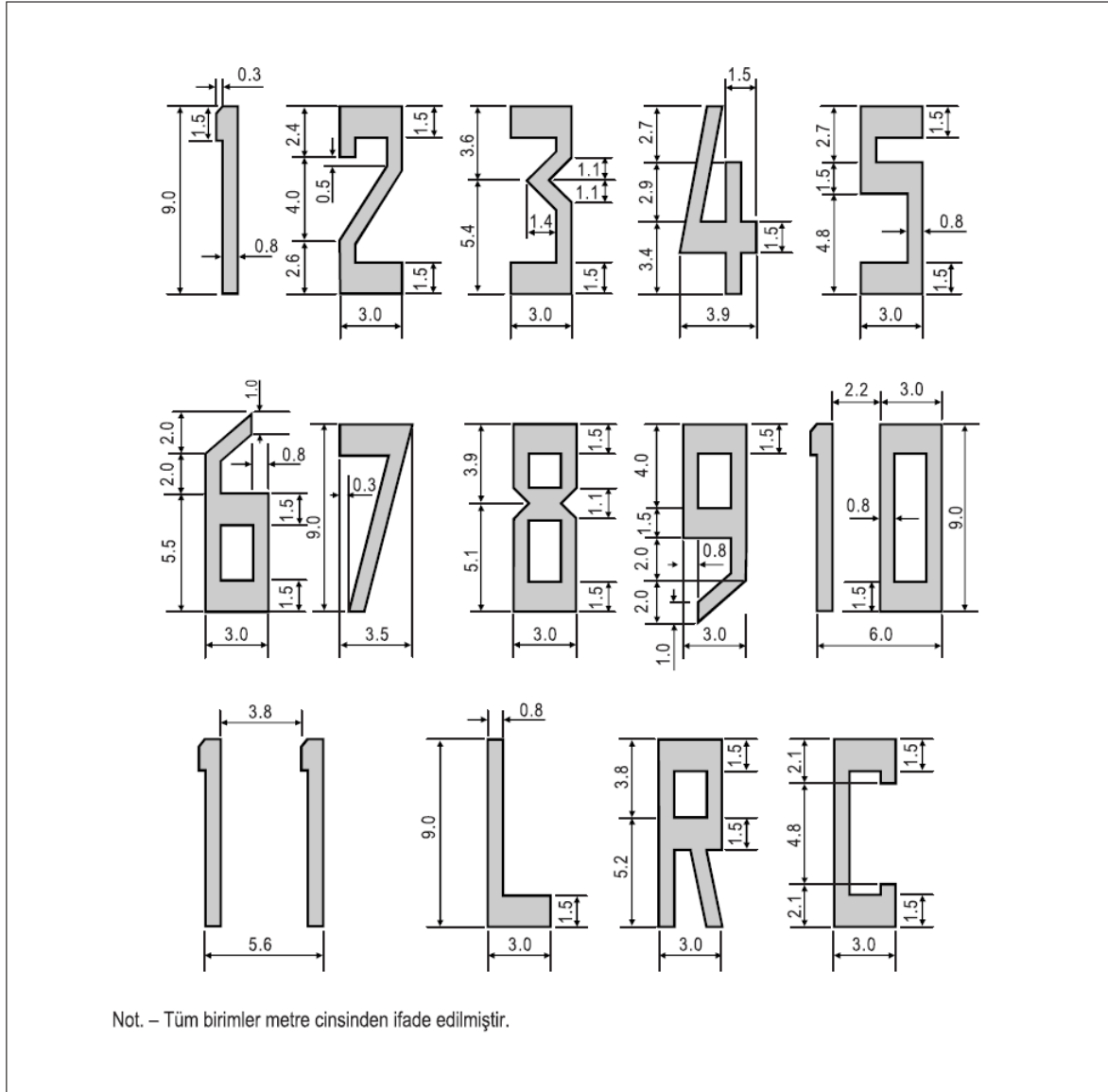
Şekil 5-3. Pist tañıtma işaretlemelerine yönelik rakamların ve harflerin şekil ve orantıları
