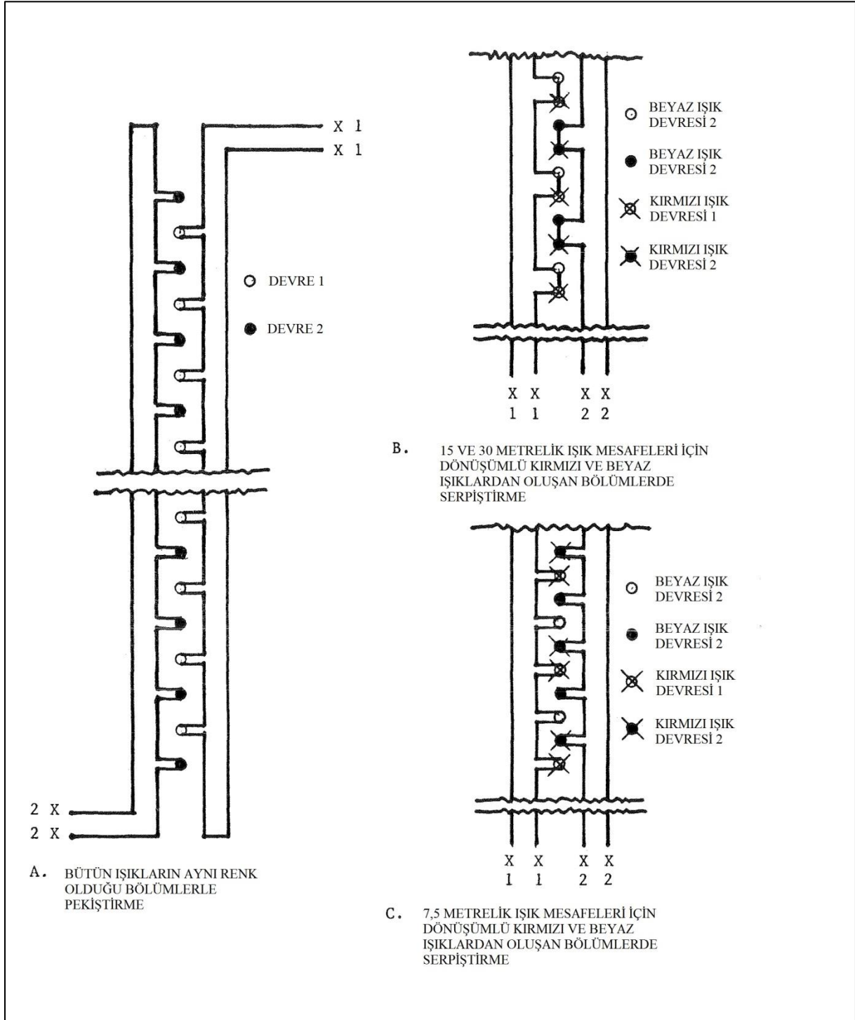
Şekil-1. Serpiştirilmiş iki devrede pist veya taxi yolu merkez hattı ışıklandırması
